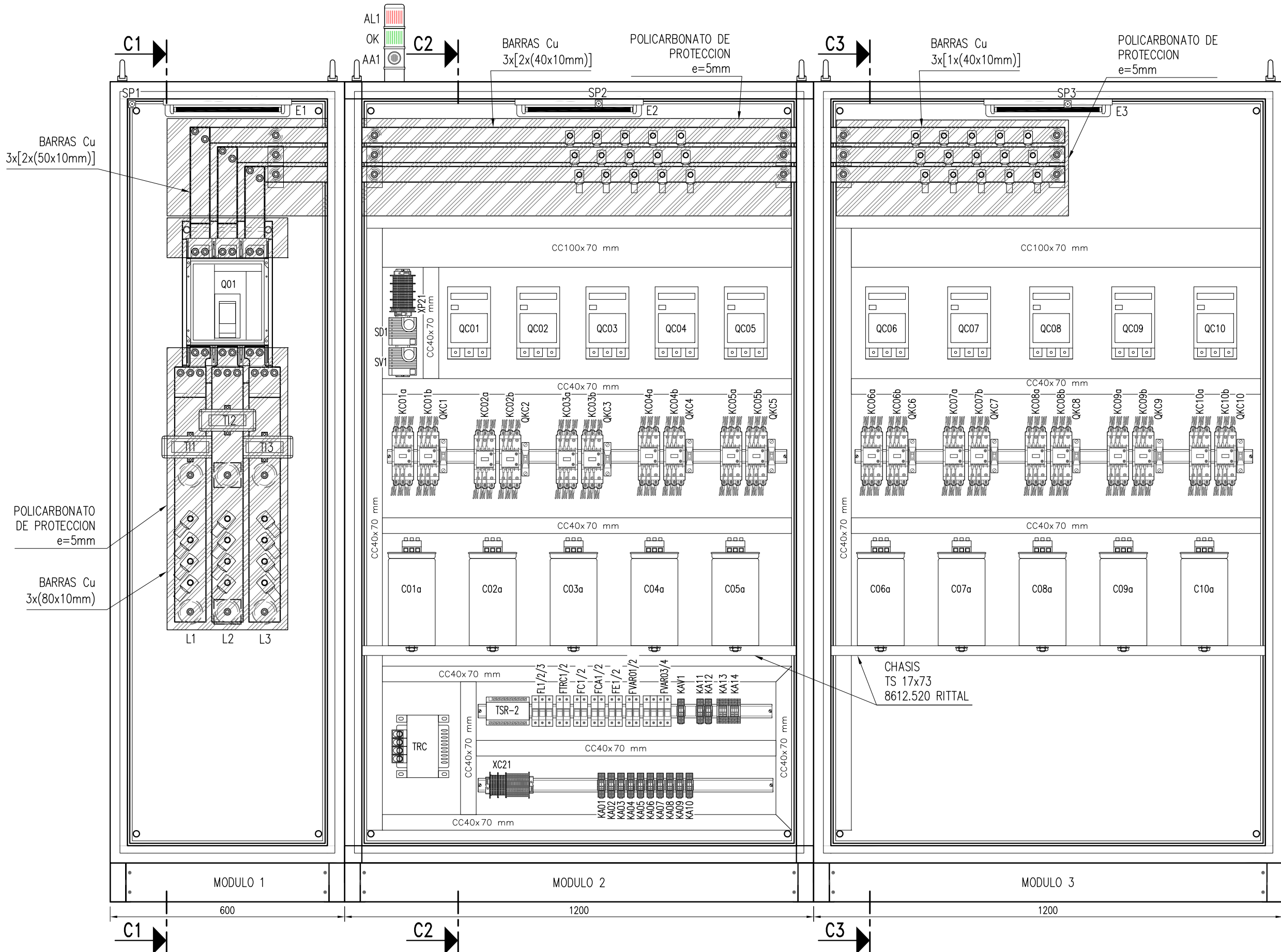
■ VISTA FRONTAL SIN PUERTA
