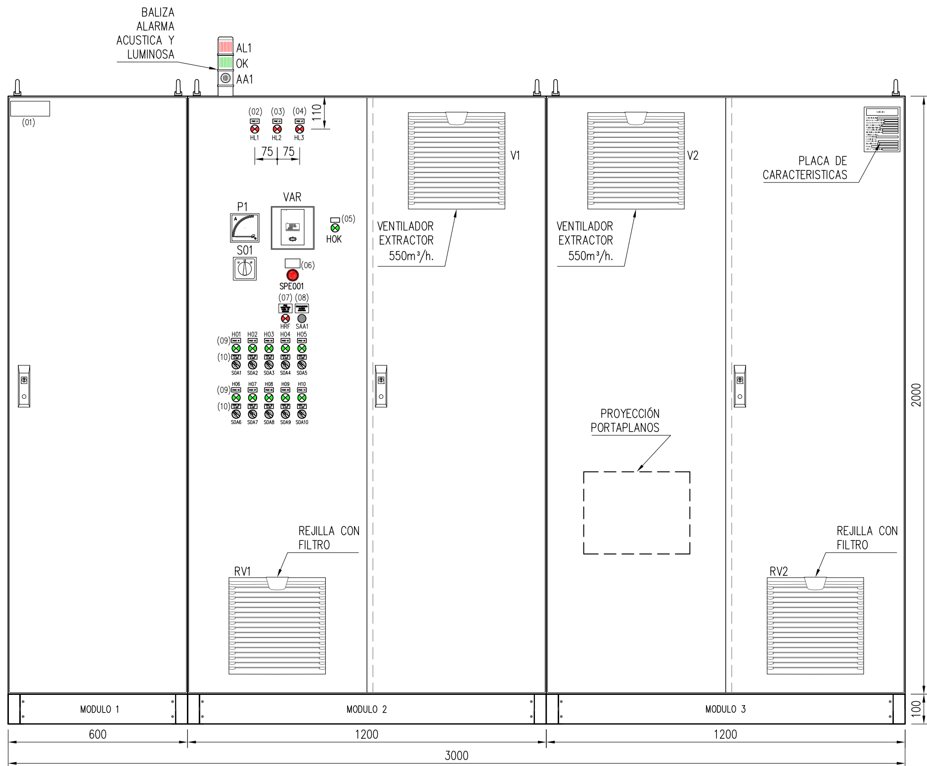
■ VISTA FRONTAL CON PUERTA
